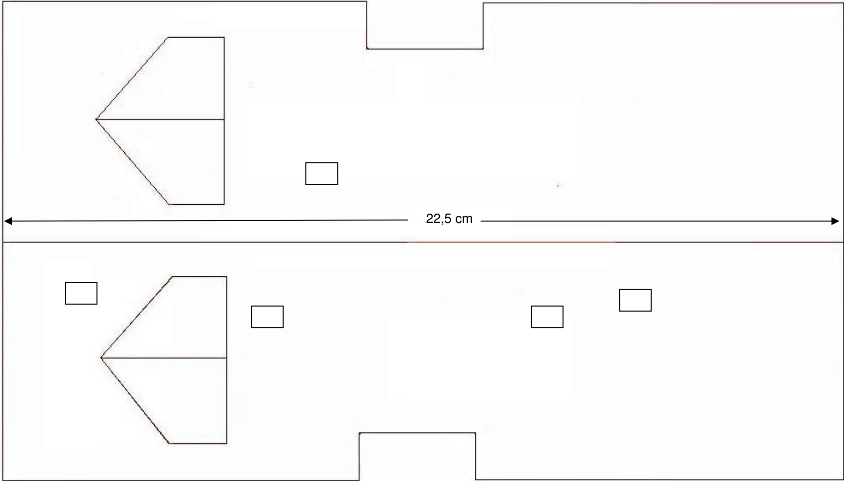
Dachschablone Hauptgebäude
